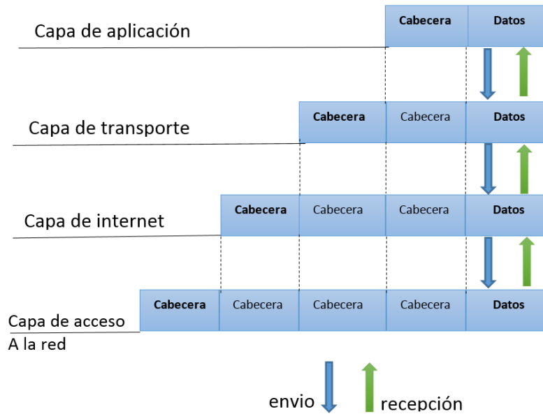
Encapsulamiento TCP/IP
