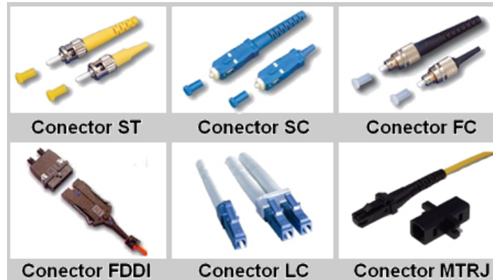
Conectores 18
