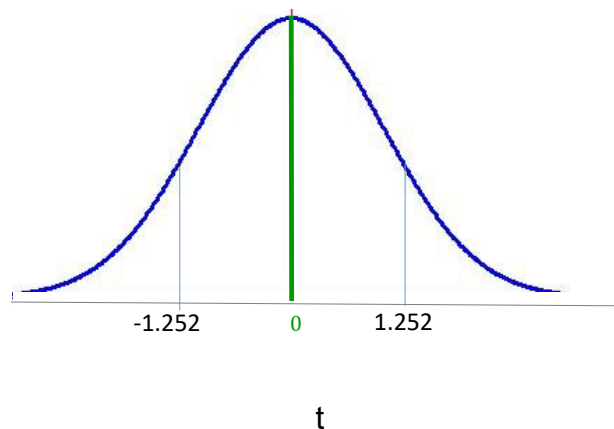
Figura 5. Segmentación de la distribución t con cuatro grados de libertad considerada en el problema
