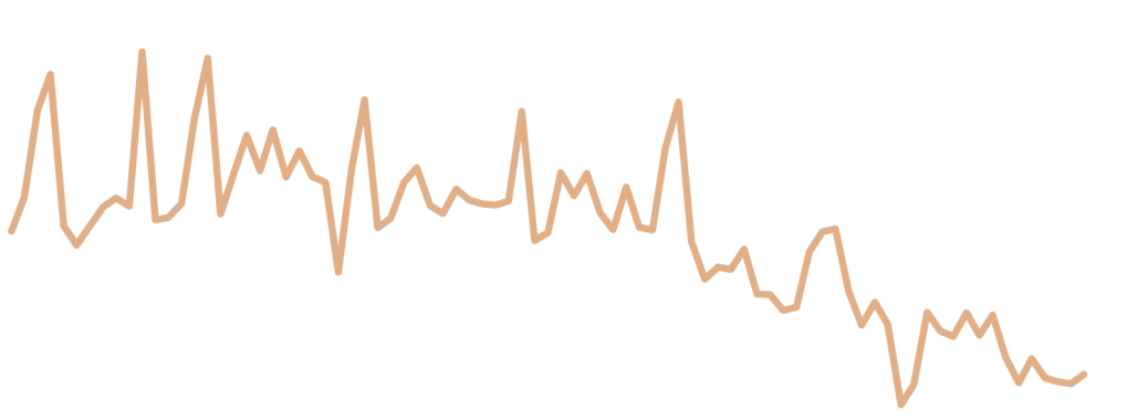
Figura 2. Serie de tiempo con tendencia negativa
