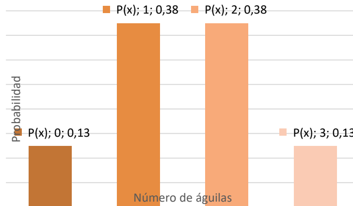
Figura 1. Distribución de probabilidades de la variable aleatoria asociada al número de águilas observadas en tres lanzamientos de una moneda de diez pesos
