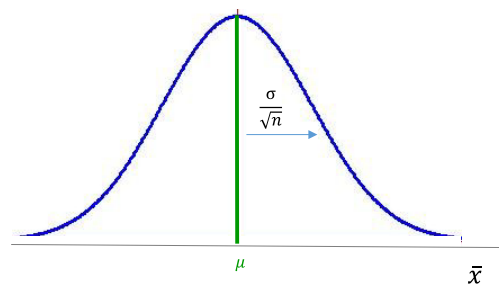
Figura 3. Distribución muestral de la media
