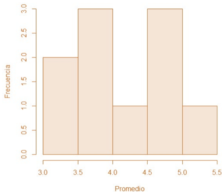
Figura 2. Distribución de frecuencias de los promedios de antigüedad de una muestra de tres empleados del área de planeación
