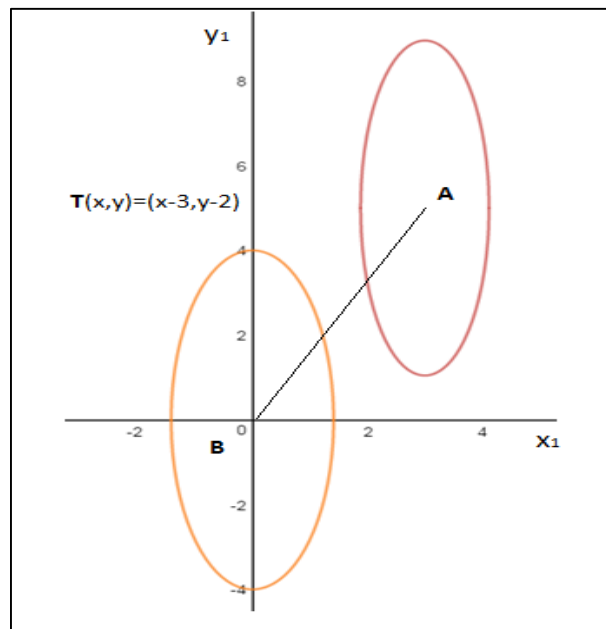
Efecto de la transformación lineal T A \rightarrow B
