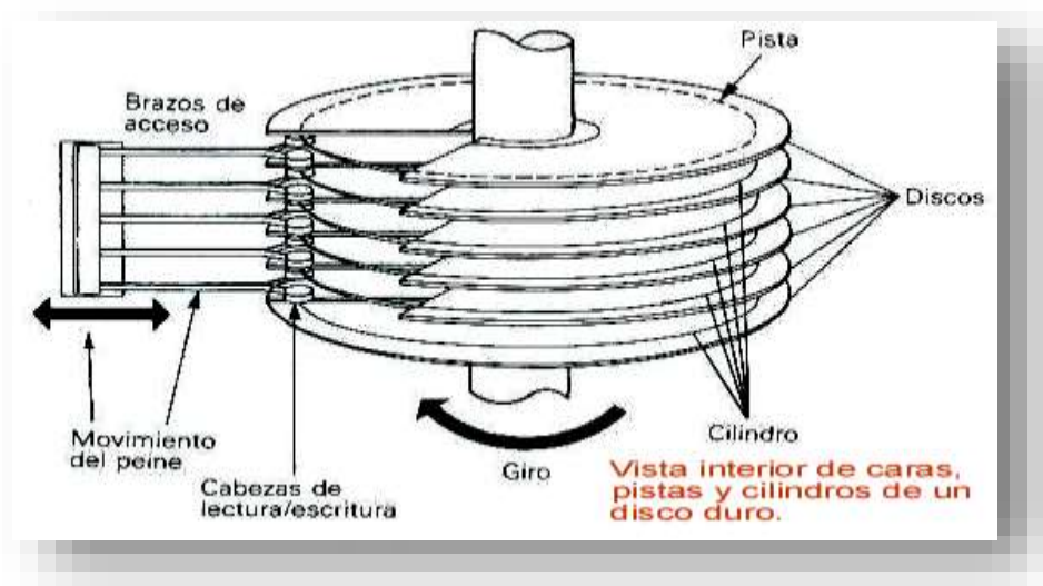
Partes y componentes de la unidad lectora del Disco duro
