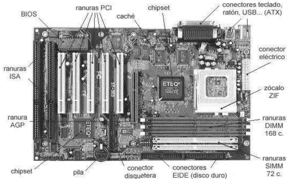
Tarjeta madre
