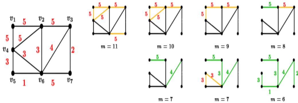
Ejemplo de aplicación del algoritmo de Kruskal 42
