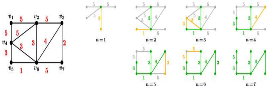
Ejemplo de la aplicación del algoritmo de Prim 43 .
