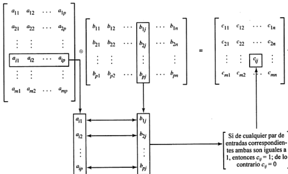
Representación gráfica de la multiplicación de matrices booleanas 34
