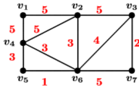
Ejemplo de grafo conexo o árbol generador 39
