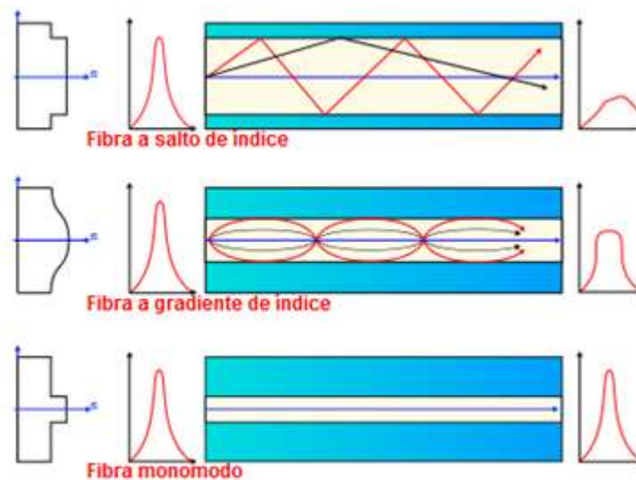
Tipos de perfiles en fibras ópticas. 16
