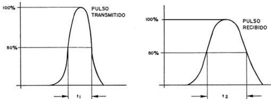
Dispersión modal 17
