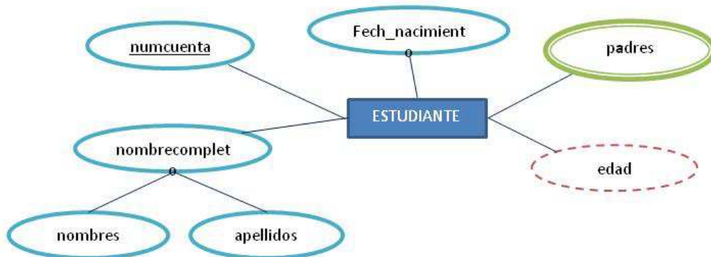
Tipos de atributos en una entidad
