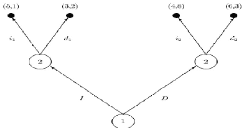
Figura 1: un juego en forma extensiva.
